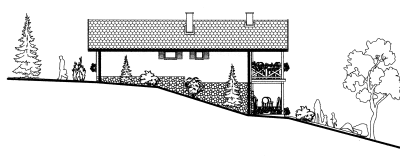
POHĽAD SEVERNÝ
