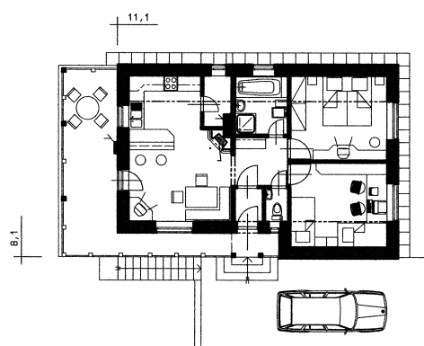
PRÍZEMIE- úžitková plocha 59,0m 2
