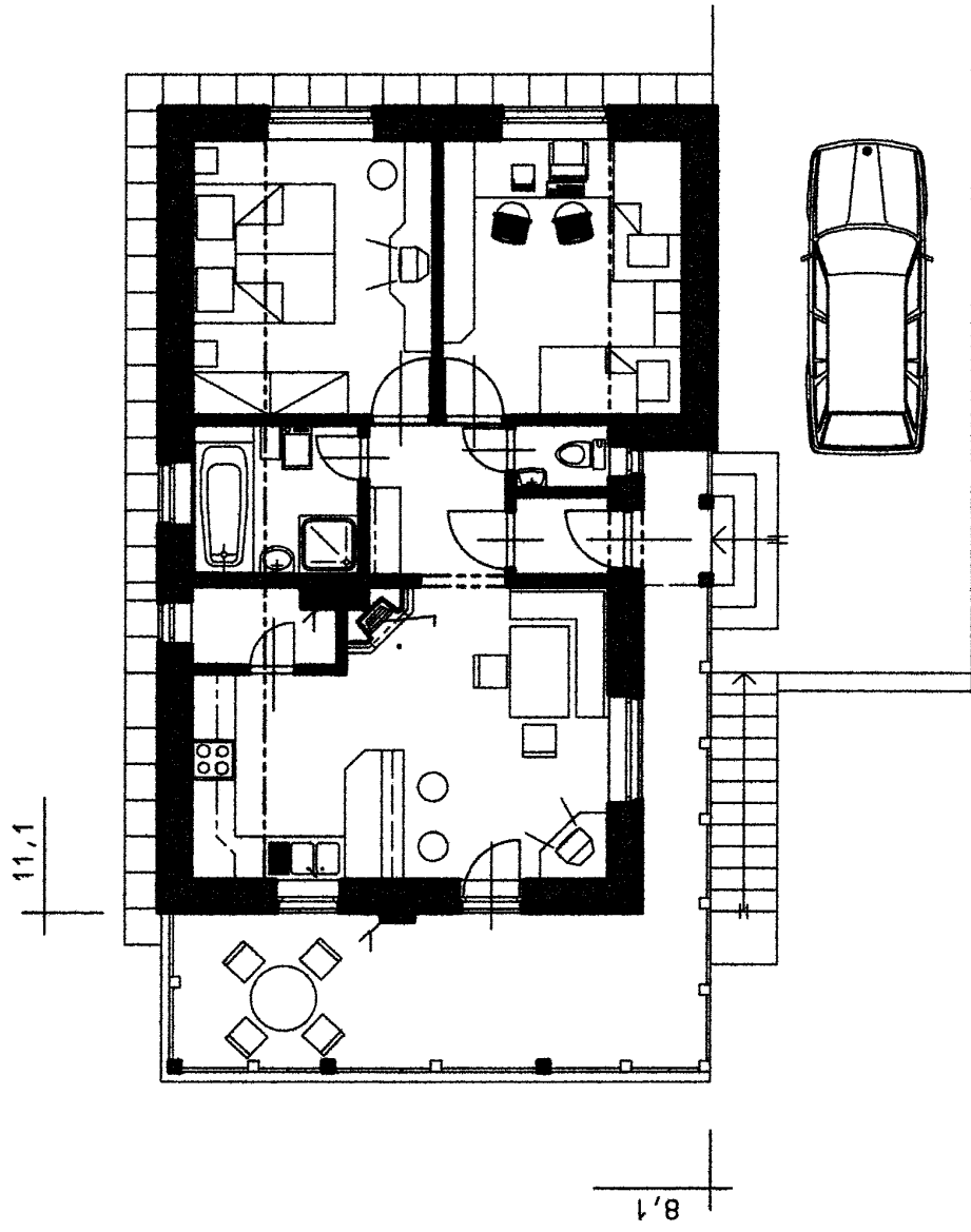
PRÍZEMIE - úžitková plocha 59,0m 2
